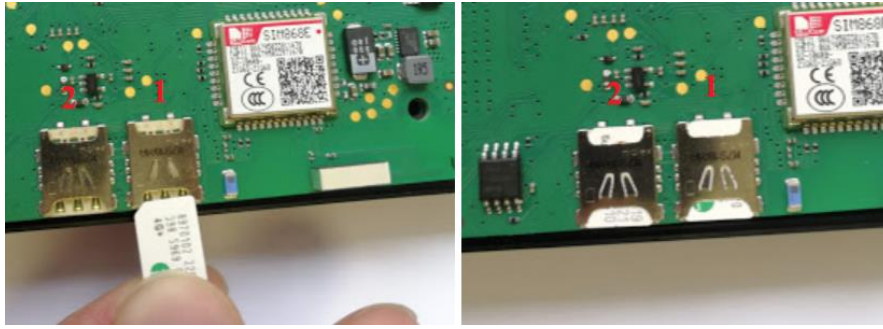
Рисунок 4.2. Установка nanoSIM-карт в терминал FORT-114M.
