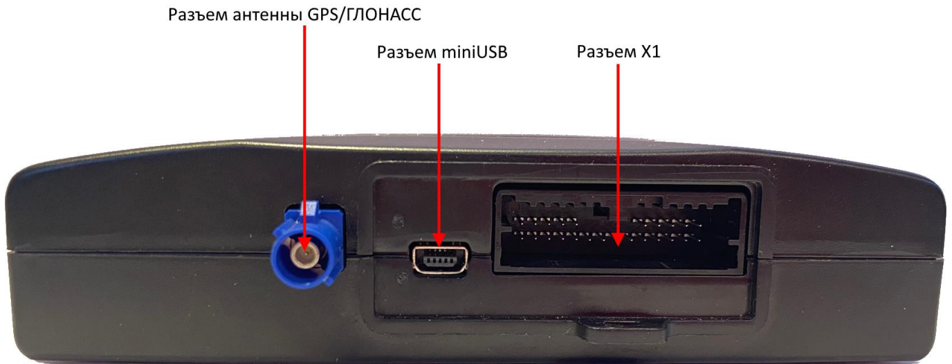
Рисунок 3.1(в) Сторона разъемов терминала FORT-114EM
